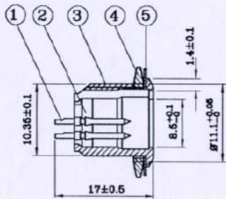
A-A SECTION
