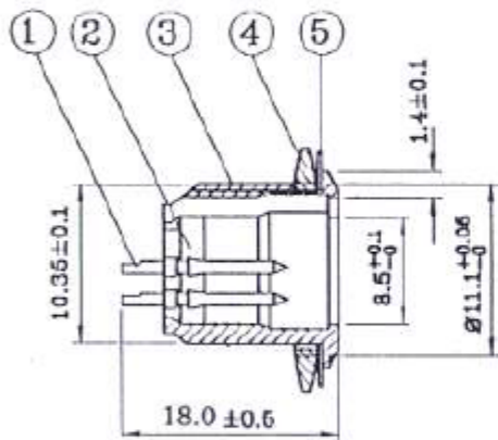
A-A SECTION
