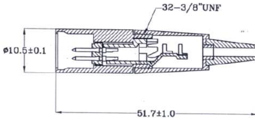
A-A SECTION
