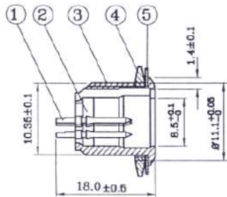
A-A SECTION
